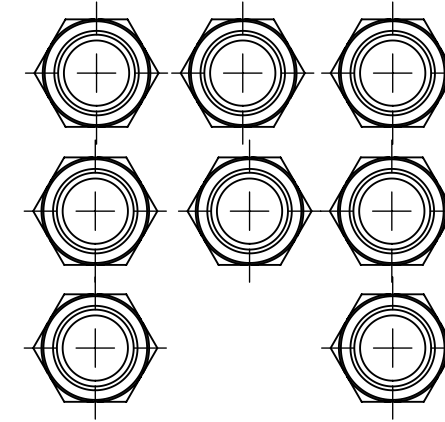
E00-3600 - 8 EA. NUT AN365-624A (3/8-24 FIBERLOCK)
